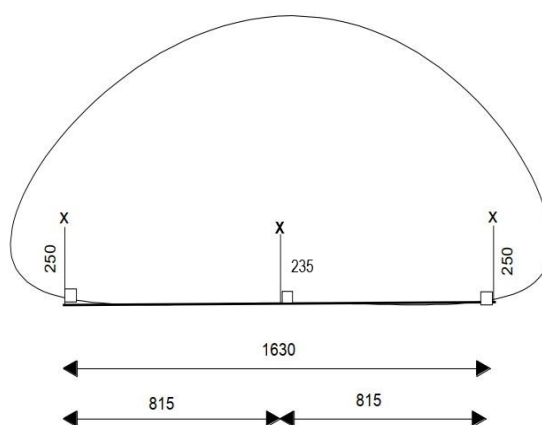
Figuur 1 Maatvoering t.b.v. van de 3 te boren gaten in het wegdek.
