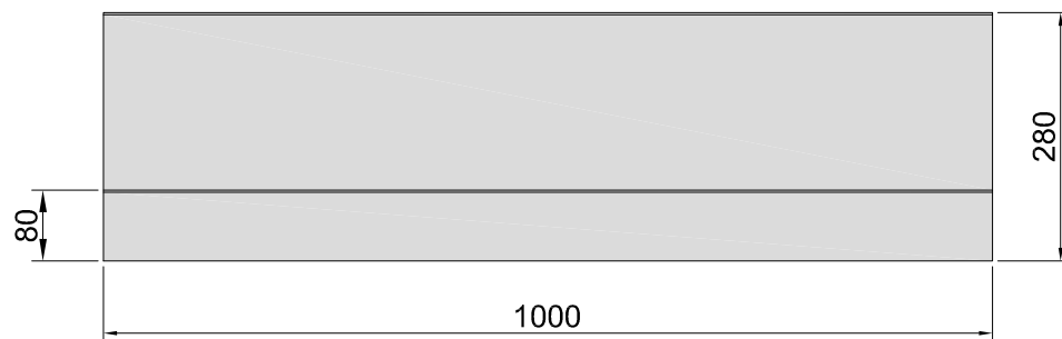
Vooraanzicht
