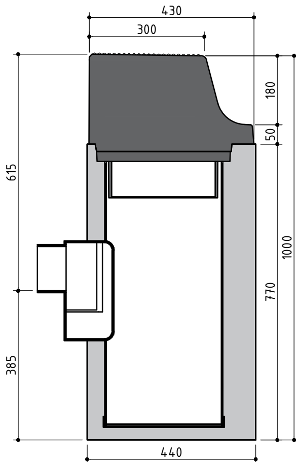
DOORSNEDE A-A
