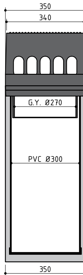
DOORSNEDE B-B
