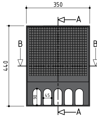
BOVENAANZICHT
